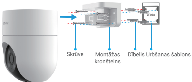
2. att. Sienas stiprinājums
