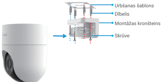
1. att. Griestu stiprinājums
